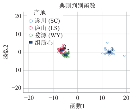
图 3 典型判别散点图
