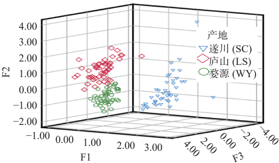
图 2 3 种主成分三维分布图
