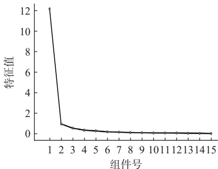
图 1 3 个县茶叶主成分碎石图
