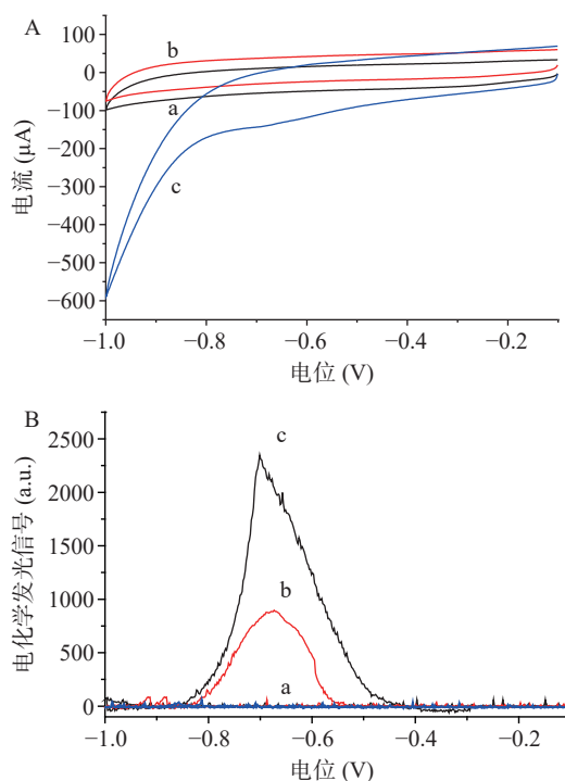
图4 不同修饰电极的循环伏安曲线图(A)与电化学发光信号—电位曲线图(B)
